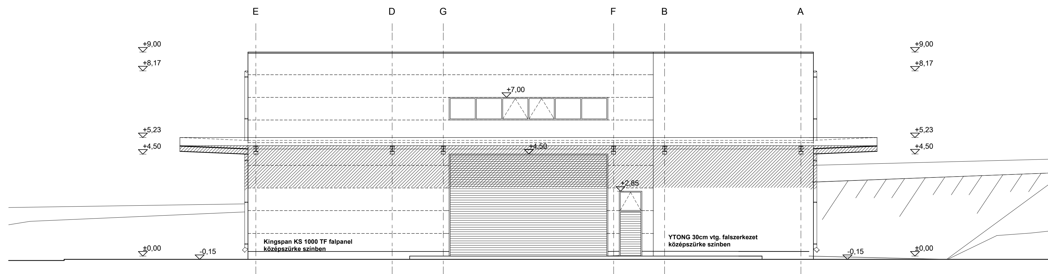
KELETI HOMLOKZAT
