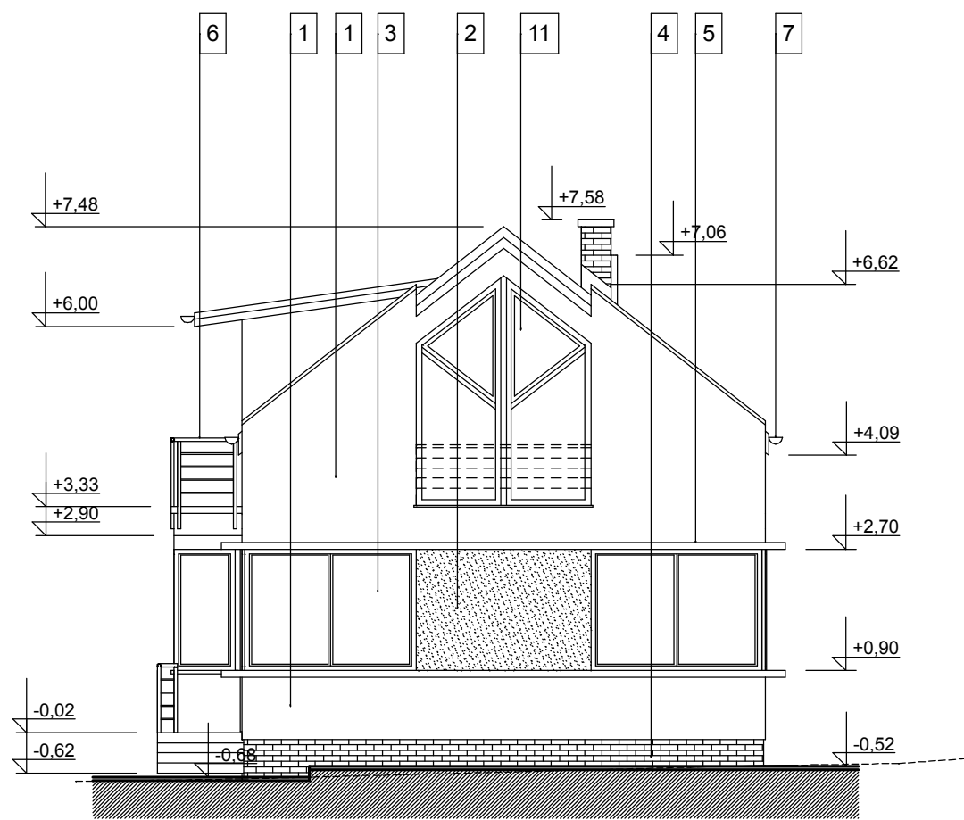
TERVEZETT DÉL-KELETI HOMLOKZAT
