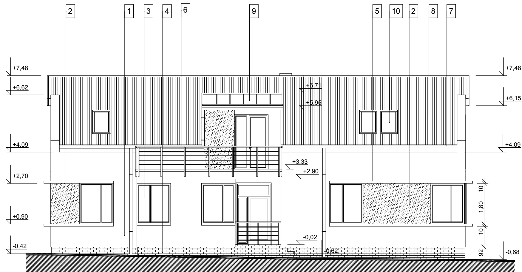
TERVEZETT DÉL-NYUGATI HOMLOKZAT
